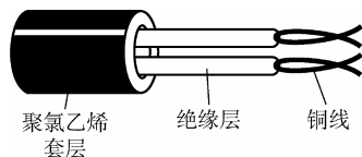
(a) 无屏蔽双绞线
