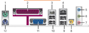
图10 编号2为电脑上的并口（并行传输），用于连接打印机、扫描仪等
