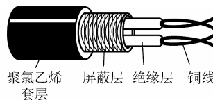
(b) 屏蔽双绞线
